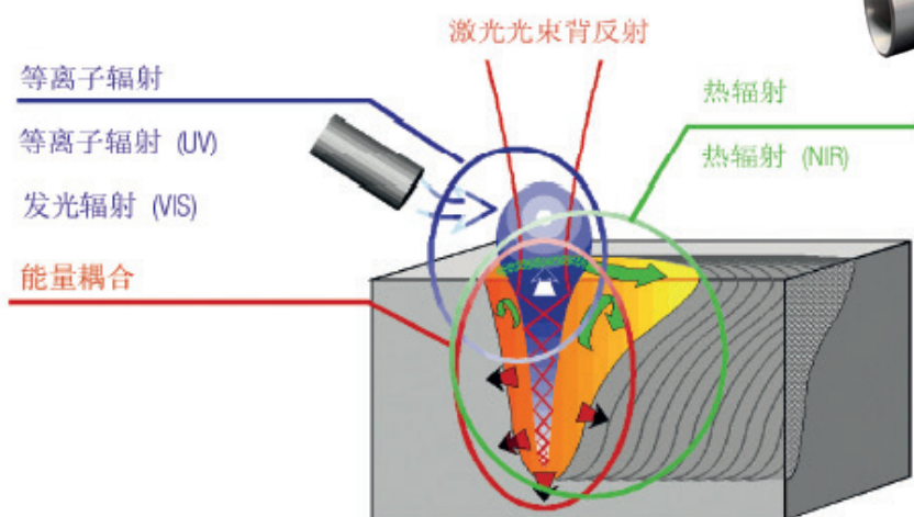
LWM检测原理 – LWM可实时获取热辐射、激光光束背反射和等离子辐射信号
